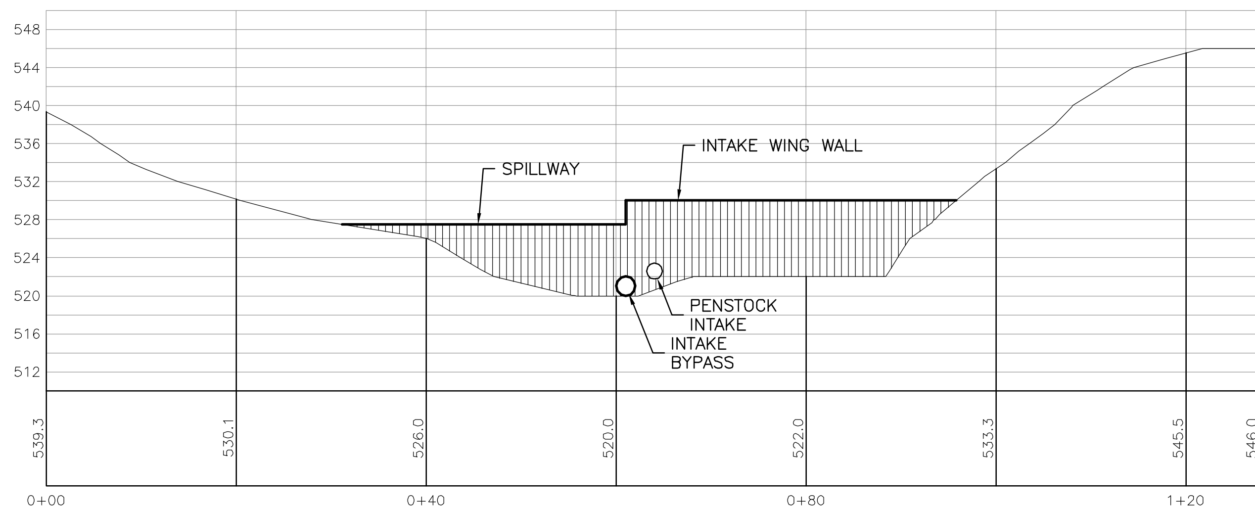
2 INTAKE ELEVATION SCALE: 1" = 10'
